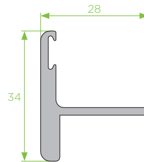
PT - 02 remate batente
