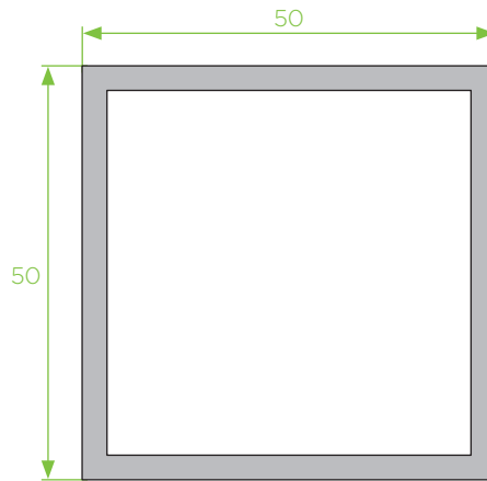
PT - 50 tubo quadrado (50x50x3,0)
