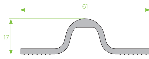
PT - 23 rail portão correr
