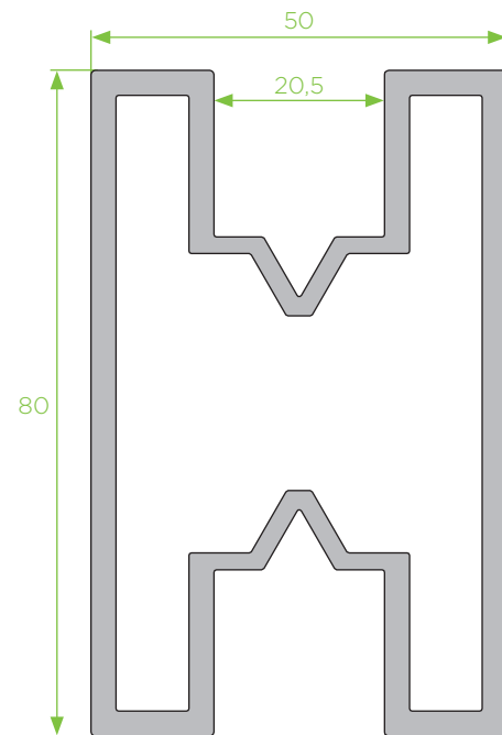
PT - 29 travessa
