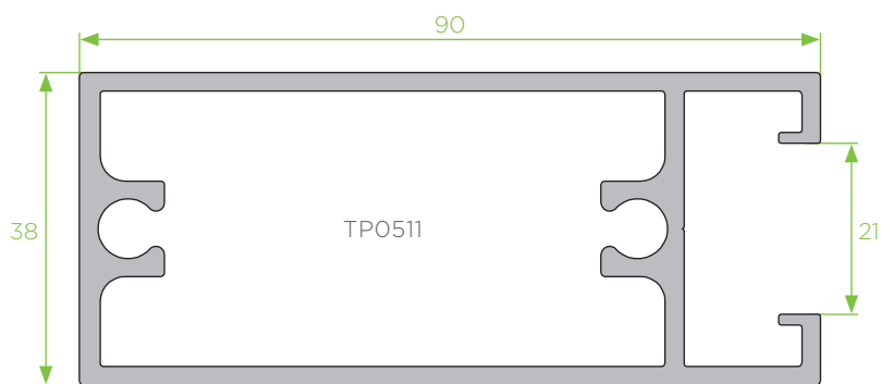
PT - 32 travessa superior/inferior
