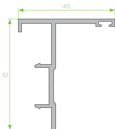
PT - 34 batente
