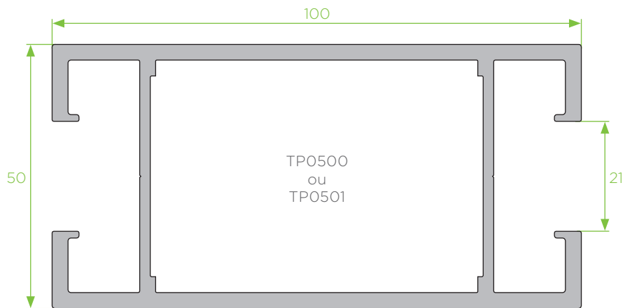
PT - 31 prumo vertical
