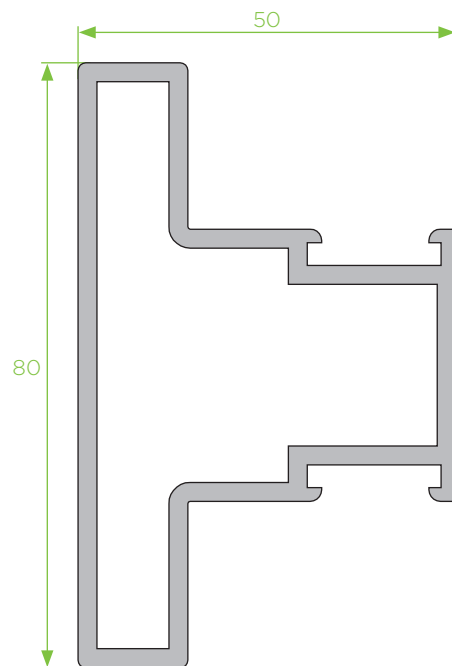
PT - 04 travessa
