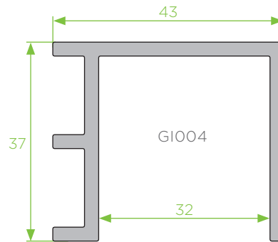
PT - 05 calha para guia correr
