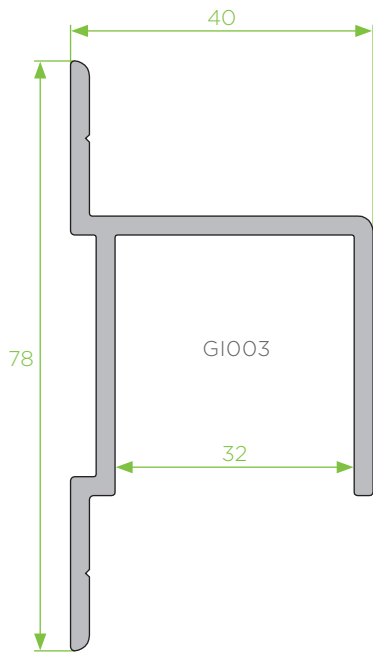
PT - 21 calha para guia correr
