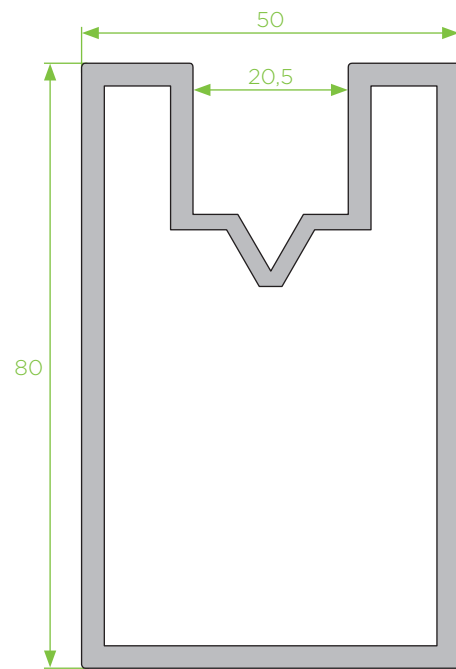
PT - 09 folha móvel
