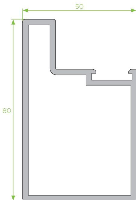
PT - 03 folha móvel
