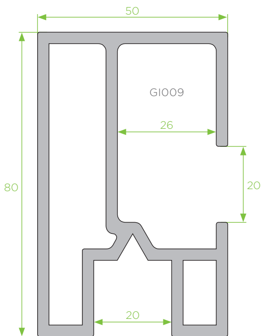
PT - 10 folha móvel
