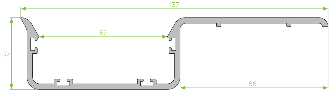
PT - 08 batente lateral correr
