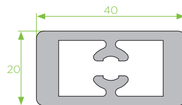
BL - 21 prumo vertical
