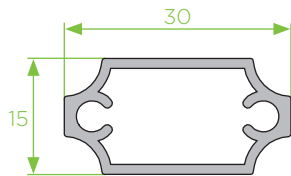
BL - 11 prumo vertical
