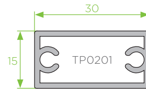
BL - 13 prumo vertical
