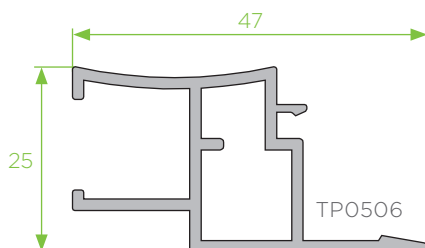
BL - 22 receptor de vidro
