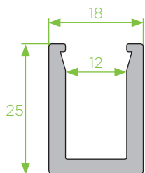
BL - 03 receptor de vidro
