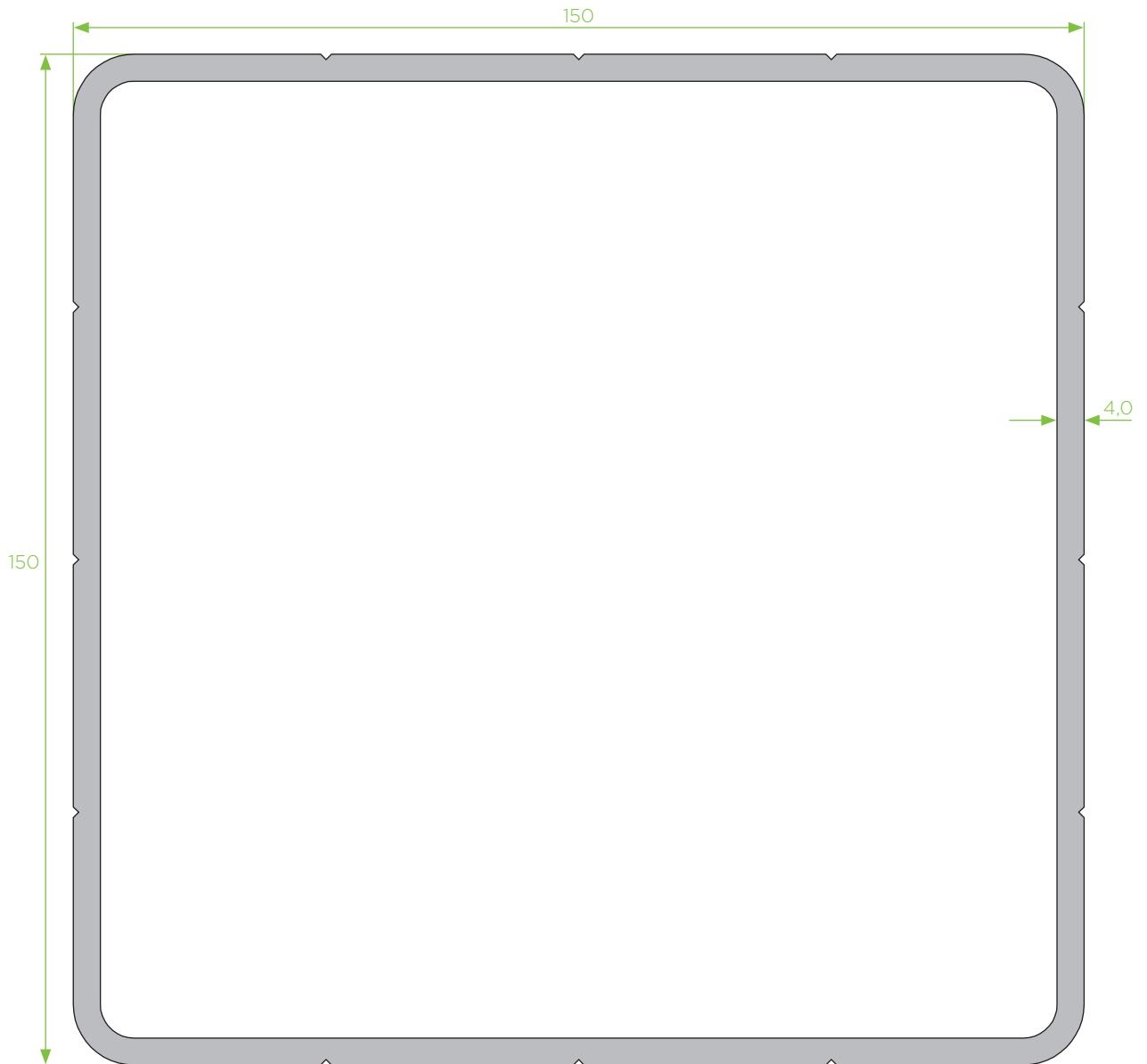
PT - 25 perfil poste 150x150x4
