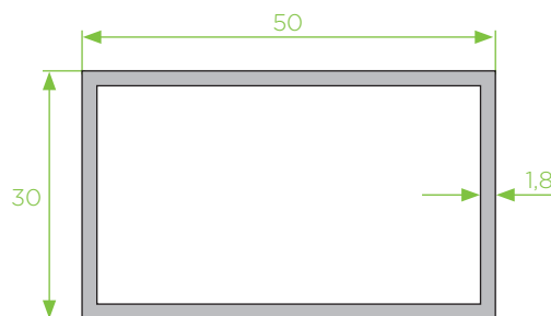
50x30x1,8 tubo retangular
