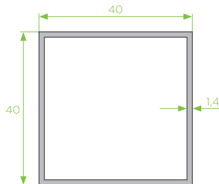
40x40x1,4 tubo quadrado
