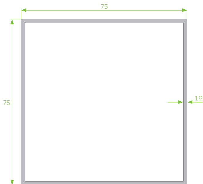
75x75x1,8 tubo quadrado
