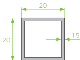
20x20x1,5 tubo quadrado
