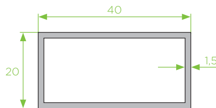
40x20x1,5 tubo retangular
