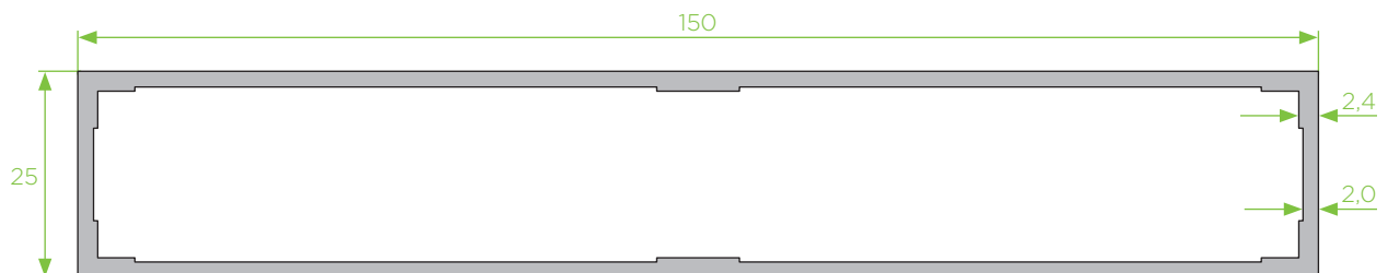
150x25x2,4 tubo retangular
