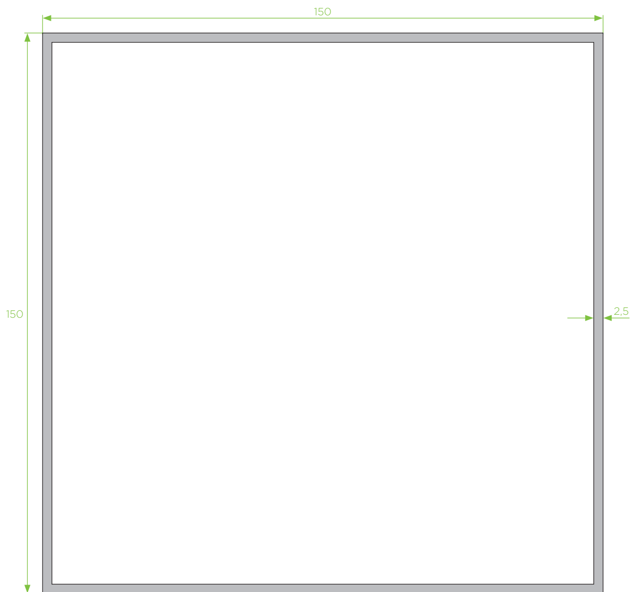
150x150x2,5 tubo quadrado
