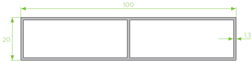
P - 30 tubo retangular com reforço
