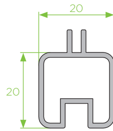
P - 71 régua de ligação
