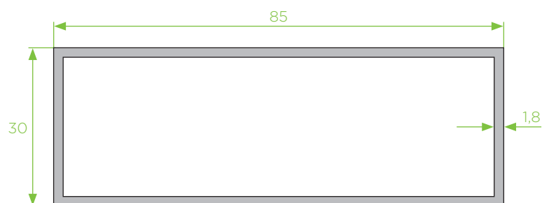
85x30x1,8 tubo retangular
