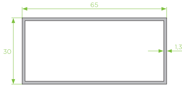
65x30x1,3 tubo retangular
