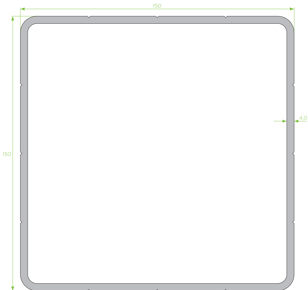
PT - 25 perfil poste 150x150x4
