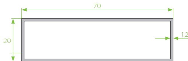
70x20x1,2 tubo retangular
