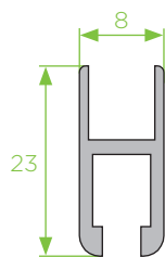
P - 32 móvel
