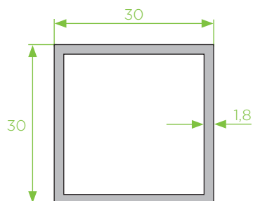
30x30x1,8 tubo quadrado
