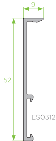
PA - 25 perfil de remate 52x9
