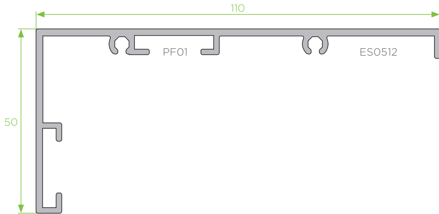
PA - 41 perfil de remate 50x110
