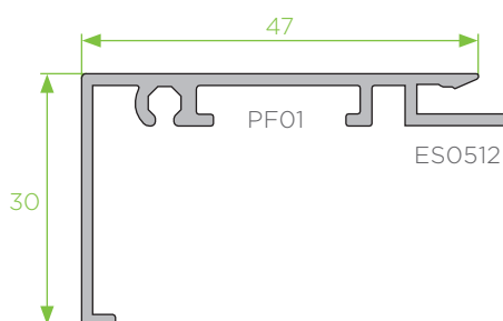
PA - 61 perfil de remate 30x47
