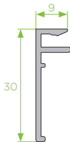
PA - 20 perfil de remate 30x9
