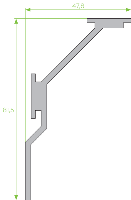
PA - 42 perfil suporte de remate
