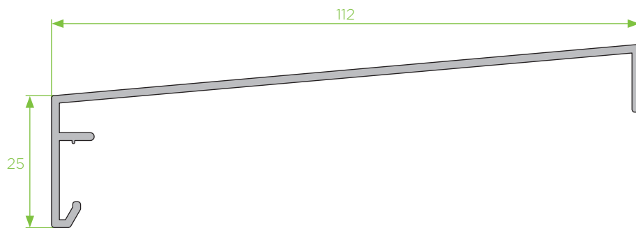
PA - 40 perfil de remate 25x112
