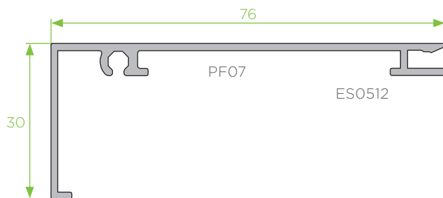
PA - 06 perfil de remate 30x76
