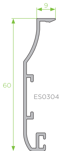
PA - 23 perfil de remate 60x9
