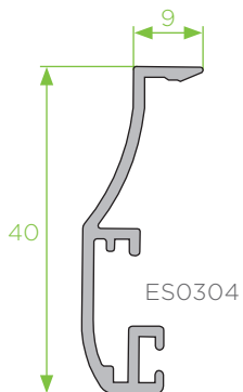
PA - 22 perfil de remate 40x9
