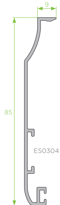
PA - 24 perfil de remate 85x9
