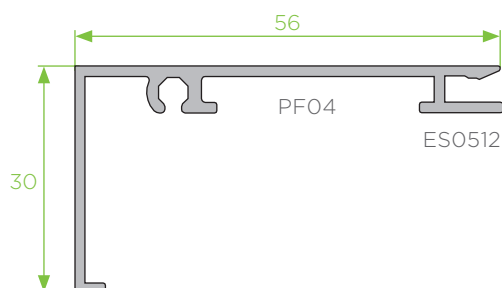
PA - 05 perfil de remate 30x56
