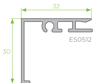
PA - 10 perfil de remate 30x32
