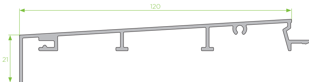
PA - 43 perfil de remate 21x120
