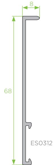
PA - 26 perfil de remate 68x8
