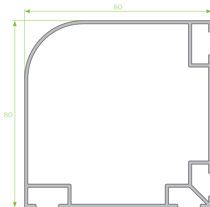
DV - 05 montante duplo
